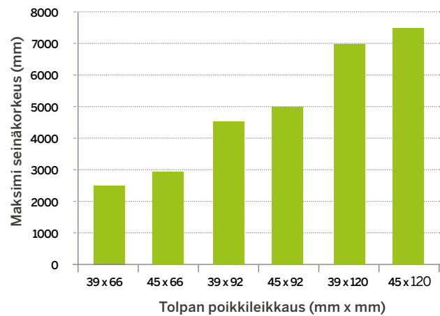
Kuva 4. Kerto-T, ei-kantavien väliseinien ohjeelliset korkeudet 600 mm tolppajaolla. Ominaiskuormana viivakuorma 0,5 kN/m 1,0 m korkeudella. Hetkellinen taipuma on w_{inst} \leq H/200 . Taulukon käyttö ei korvaa kohdekohtaista rakennesuunnittelua.
